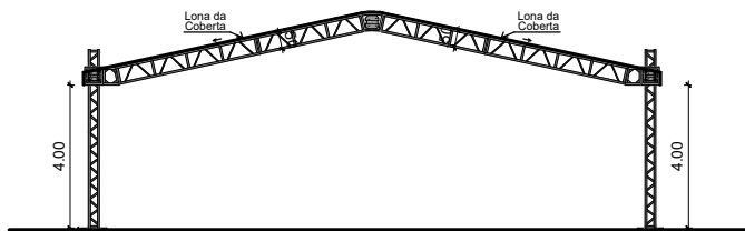
ELEVAÇÃO MARQUISE ESCALA 1/100
