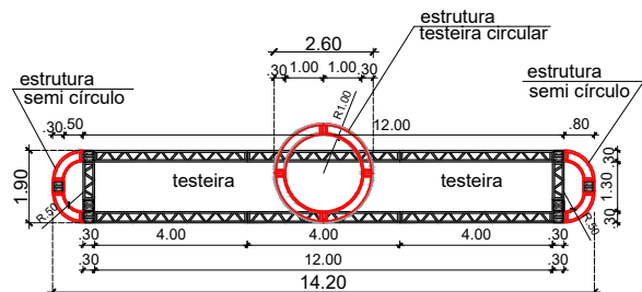
DETALHE ESTRUTURA DA TESTEIRA
