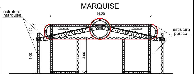
CORTE ESQUEMÁTICO MARQUISE E PÓRTICO ESCALA 1/100
