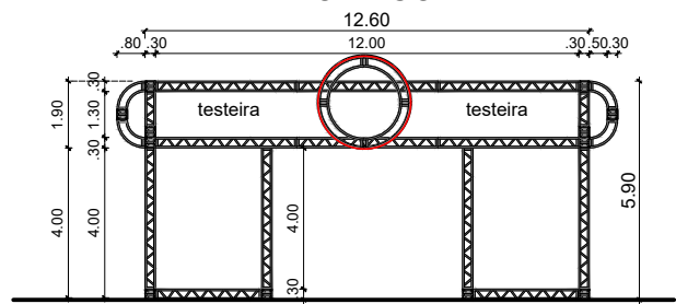
ELEVAÇÃO PÓRTICO ESCALA 1/100
