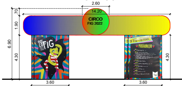
ELEVAÇÃO FRONTAL ESCALA 1/100
