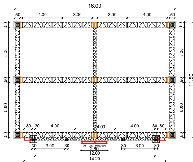
PLANTA BAIXA MARQUISE ESCALA 1/100
