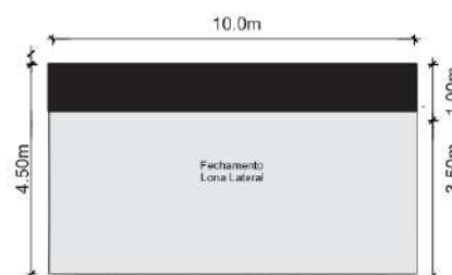
CORTE A-A' escala 1/100
